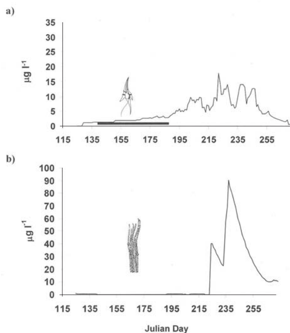
Figure 5. (a) Simulated temporal dynamics of Ceratium hirundinella in El Gergal reservoir if the water transfer from La Minilla reservoir was developed after the occurrence of the Ceratium bloom. (b) The same scenario for Aphanizomenon flos-aquae biomass ( \mu\text{g l}^{-1} ). (a) Simulación de la dinámica temporal de Ceratium hirundinella en El Gergal considerando que el trasvase de agua se hubiera efectuado tras la desaparición del bloom de Ceratium hirundinella en La Minilla. (b) El mismo escenario para la biomasa de Aphanizomenon flos-aquae ( \mu\text{g l}^{-1} ).
