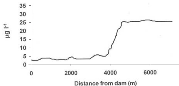
Figure 4. Longitudinal transect showing the horizontal distribution of Ceratium hirundinella biomass (expressed as chlorophyll- a content, \mu\text{g l}^{-1} ) in El Gergal reservoir following the water transfer from La Minilla. Distribución horizontal de la biomasa de Ceratium hirundinella (expresada como concentración de clorofila-a, \mu\text{g l}^{-1} ) a lo largo de un transecto longitudinal en el embalse de El Gergal tras efectuarse el trasvase de aguas desde La Minilla.
