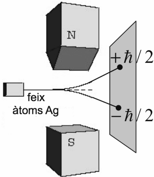
Figura 1.2: Experiment destructiu de Stern-Gerlach
